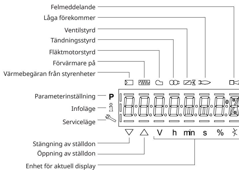
Bild 4: Displaybeskrivning
